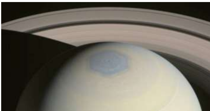
Hexadiagonaal stormpatroon boven de noordpool van Saturnus.
